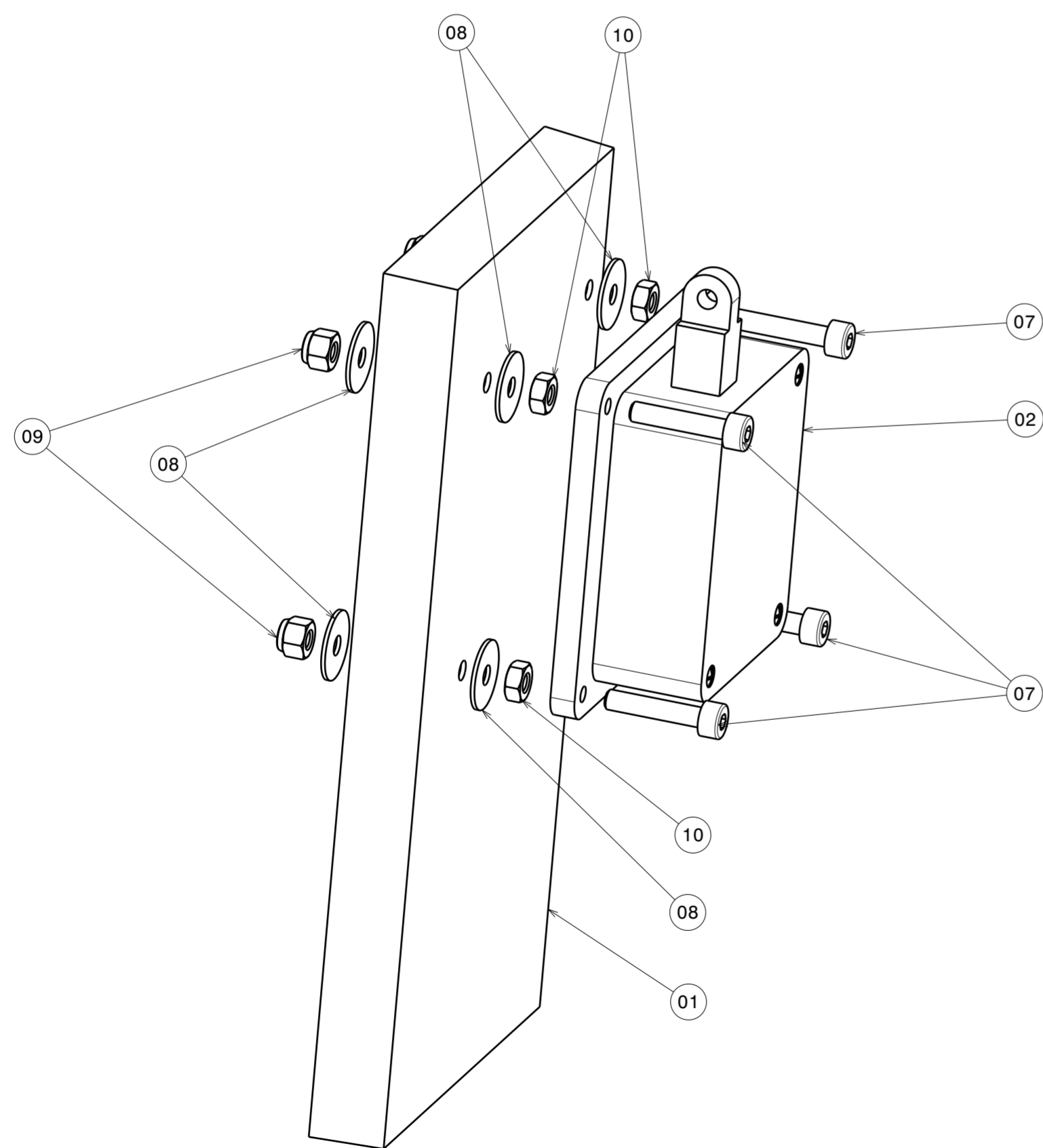
FIXATION SERVO TRIM PROFONDEUR
